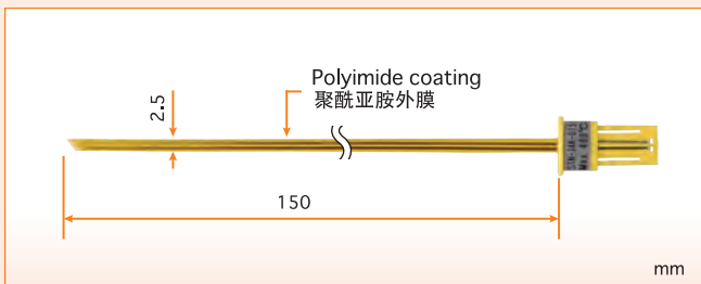
Type E model : STN-34E-015 Type K model : STN-34K-015
