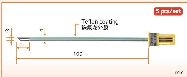
Type E model : STN-11E-010 Type K model : STN-11K-010
